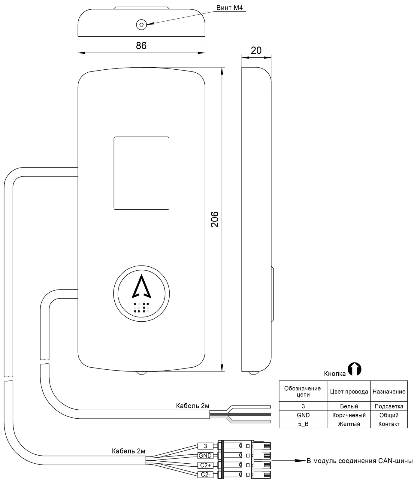
Рис.1 Внешний вид, габаритные и установочные размеры Вызывного поста ВП-1101-1086-07
